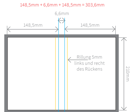
Abb. 1) Beispiel Zeitung A5: Cover mit errechneter Rückenbreite von 6,6mm ■ Überfüller
